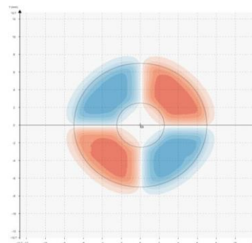
Magnetisierung Rückseite
